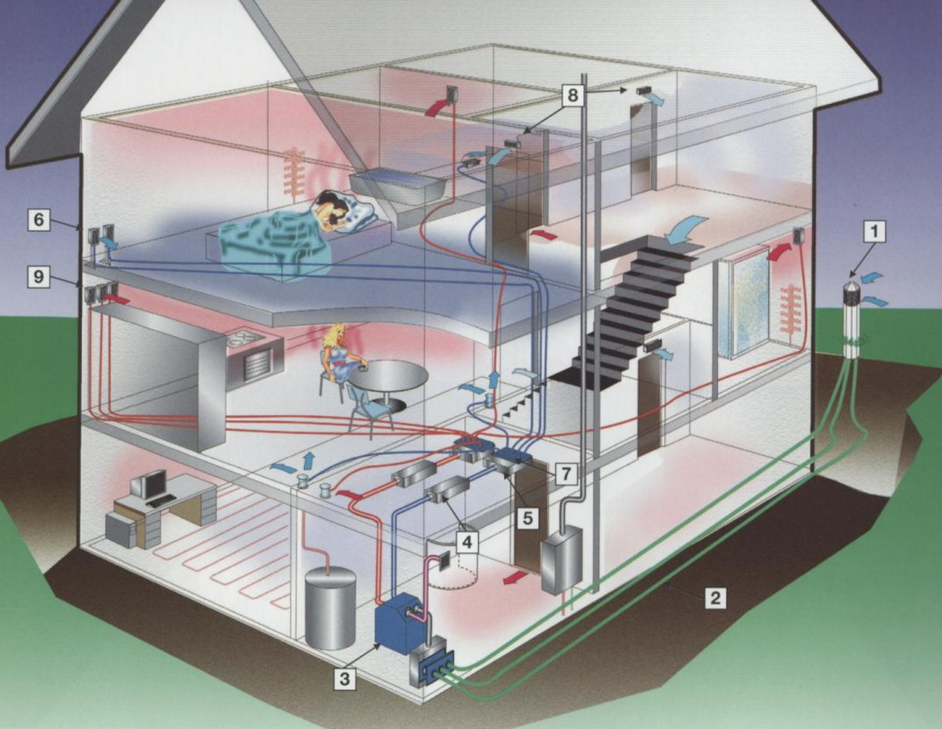
Luftverteilung Zehnder Comfofresh, Komplettsystem für die komfortable Raumlüftung.
